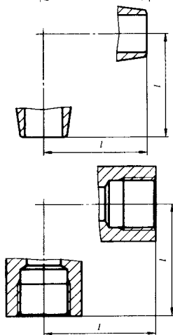
图 2 角式阀门结构长度
