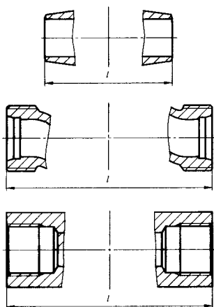
图 1 直通式阀门结构长度
